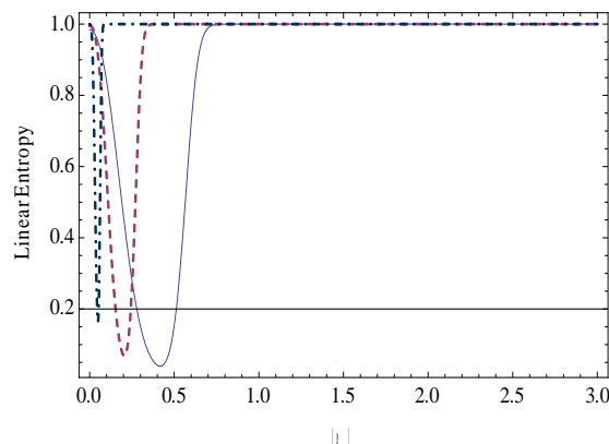
شکل ۱: آنتروپی خطی بر حسب |\alpha| برای حالت‌های همدوس پنسون سولومون برای k=3 (خط توپر)، k=4 (خط چین)، k=6 (خط-نقطه).
