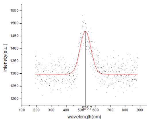
شکل ۵: طیف الکترومینیسانس دیود نورگسیل سبز
