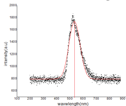
شکل ۸: طیف الکترو لومینسانس دیود نورگسیل سبز
