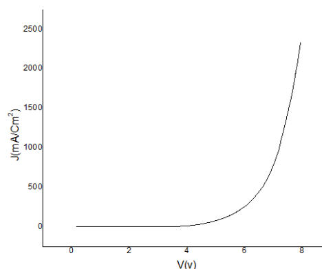
شکل ۷: نمودار ولتاژ- جریان دیود نورگسیل سبز
