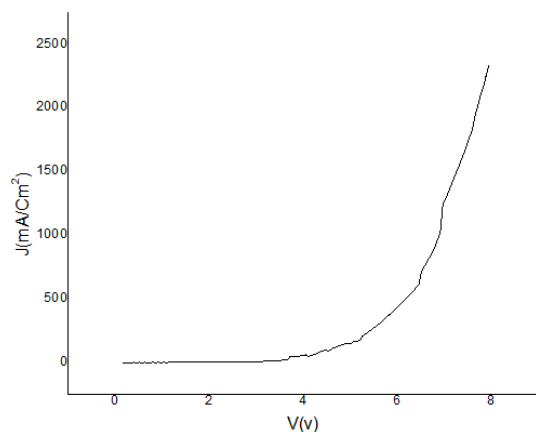
شکل ۴: نمودار ولتاژ-جریان دیود نورگسیل سبز
