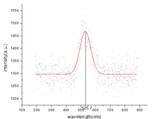
شکل ۵: طیف الکترومغناطیس دیود نورگسیل سبز
