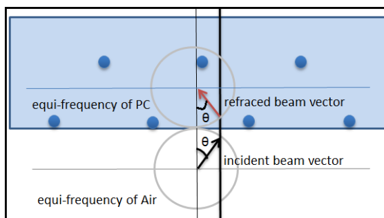
شکل ۳: نمودار کانتور هم‌فرکانس بلور فوتونی مثلثی و هوا در فرکانس \frac{0.222}{a} \times 2\pi c . هر دو نمودار باهم یکسانند. زاویه ورودی و شکست \theta باهم برابر است.
