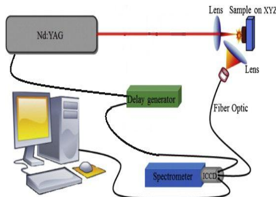
شکل ۱: چیدمان آزمایش
