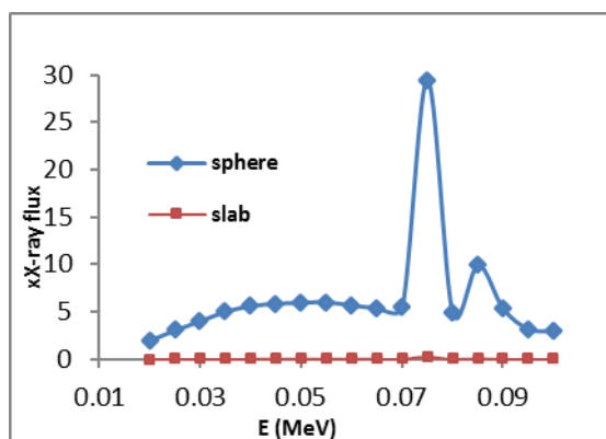
شکل ۵: مقایسه دو هدف تیغه ای و کروی در t=d=100\mu\text{m} . همچنین نتایج شبیه سازی ها برای هدف سربی با شکل نیم کره و کره ناقص تحت بررسی می باشند.
