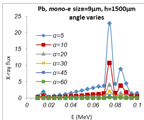
شکل ۱ ب مقایسه هدف مخروطی شکل با زاویه راس های مختلف در ارتفاع ۱۵۰۰ میکرومتر
