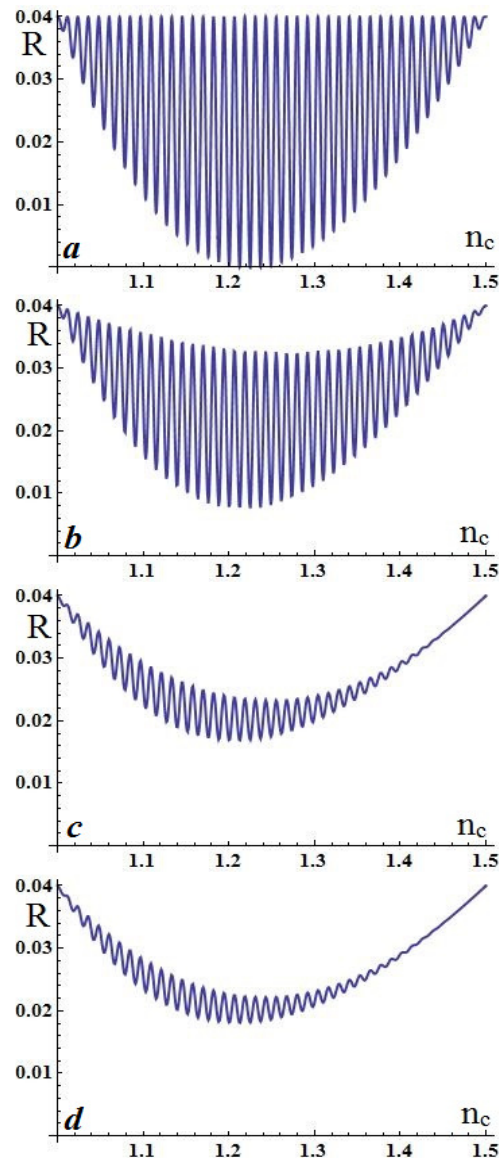
شکل ۲: ضریب بازتاب پوشش ضدبازتاب بر حسب ضریب شکست آن با ضخامت ثابت پوشش و نور همدوس (a)؛ با افت‌وخیز ضخامت پوشش ولی نور همدوس (b)؛ با ضخامت ثابت پوشش ولی نور ناهمدوس (c)، و افت‌وخیز ضخامت به همراه نور ناهمدوس (d).
