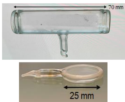
شکل ۱: از بالا سلول مرجع با ابعاد 70 \times 25 ، و سلول میلیمتری با ابعاد 20 \times 3 میلی‌متر.
