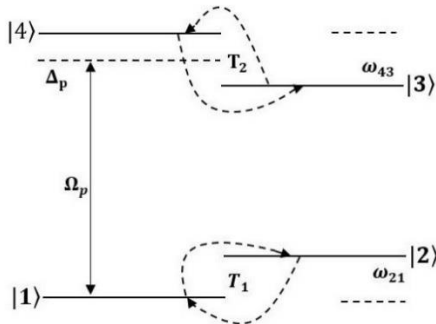
شکل ۱: سطح انرژی سامانه‌ی چهارترازی دوگانه [۶]
