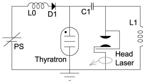
شکل ۲- مدار الکتریکی لیزر با تاپروترون
