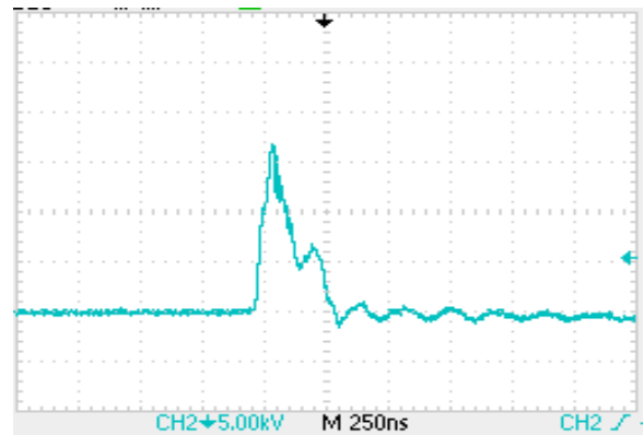
شکل ۶- تپ ولتاژ اعمال شده به لیزر با استفاده از تایروترون
