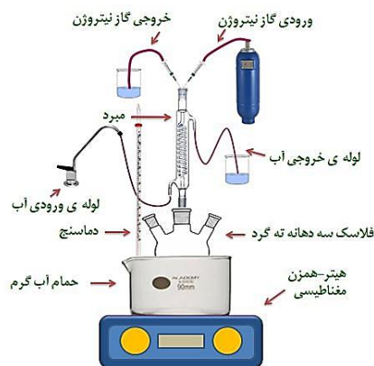
شکل ۱: شماتیک رآکتور استفاده شده جهت ساخت میکروکرات پلیمری.
