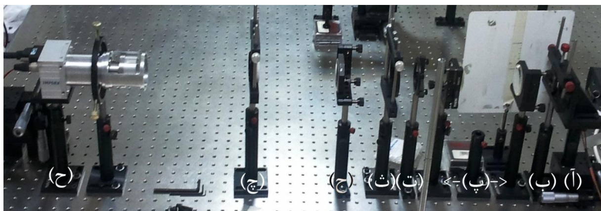
شکل ۵: چینش موازی ساز به همراه دوربین (لنز و CCD) - (آ) LED، (ب) گشودگی اولیه، (پ) لنزهای 4f، (ت) Pin Hole، (ث) گشودگی پرتوی خروجی، (ج) عدسی موازی کننده خروجی، (چ) فیلتر شدتی ND Filter، (د) CCD و لنز قابل جابجایی.
