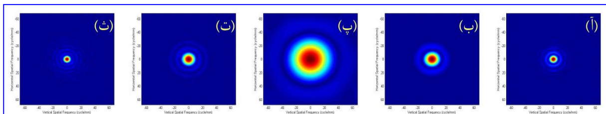
شکل ۴: MTF دو بُعدی در - (آ) وضعیت اول \theta = 0^\circ ، (ب) وضعیت دوم \theta = 120^\circ ، (پ) وضعیت سوم \theta = 240^\circ ، (ت) وضعیت چهارم \theta = 360^\circ ، (ث) وضعیت پنجم \theta = 480^\circ (قرمز بیشینه، آبی کمینه).
