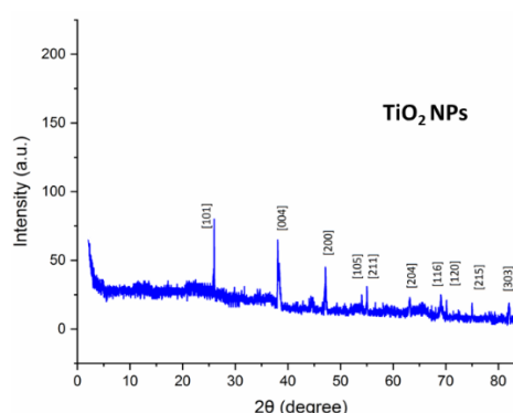
شکل ۱: الگوی پراش پرتو X نانو ذرات \text{TiO}_2
