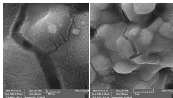
شکل ۱ تصاویر SEM ساختار پروسکایت سنتز شده به روش کوره دمای ۱۲۰ درجه سانتی گراد
