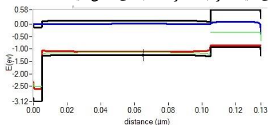
شکل ۲. نمودار ساختار باندی لایه های مختلف سلول خورشیدی آلی مورد مطالعه.
