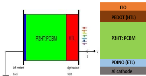
شکل ۱. ساختار شماتیک سلول خورشیدی آلی ناهمگن توده ای مورد مطالعه.
