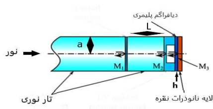
شکل ۱: شماطیک تداخل سنج فابری-پرو دیافراگمی
