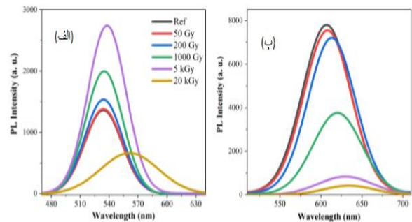
شکل ۴. الف) طیف نوری تابش قبل و بعد از قرار گرفتن در معرض گاما برای (ب) CdTe/CdSe/CdS و CdTe
