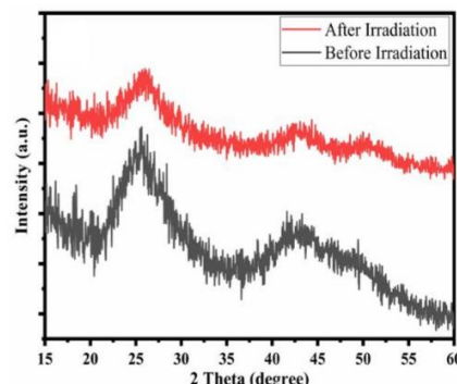
شکل ۴: الگوی XRD نقاط کوانتومی \text{CdTe/CdSe/CdS} قبل و بعد از تابش گاما
