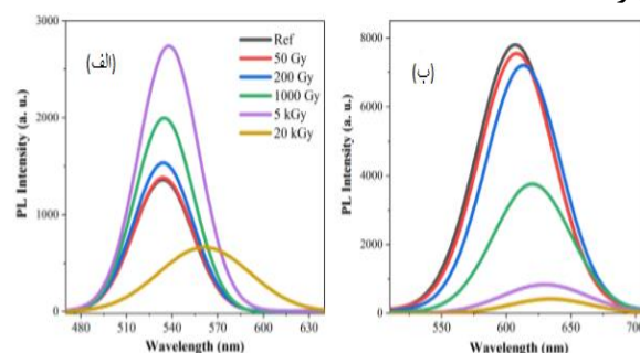
شکل ۴. الف) طیف نورتابی قبل و بعد از قرار گرفتن در معرض گاما برای (ب) \text{CdTe/CdSe/CdS} و \text{CdTe}
