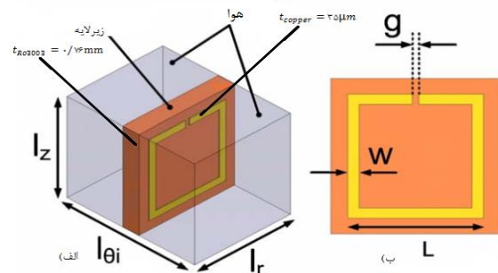
شکل ۳: طرحواره الف) سه بعدی. ب) دوبعدی سلول واحد پیشنهادی با مشخصات g = 0.18(mm) و l_{0i} = 6(mm) ، L_x = L_y = 4/5(mm) ، L_z = 3/6(mm) و W = 0.3(mm) زیر لایه از جنس RO3003 با ضخامت t_{R03003} = 0.76mm و مشدد حلقوی شکافدار از جنس مس با ضخامت t_{copper} = 35\mu m می باشد.
