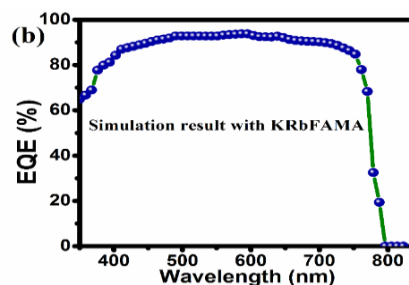
شکل ۲: الف) شبیه‌سازی منحنی چگالی جریان-ولتاژ و ب) شبیه‌سازی منحنی بازده کوانتوم خارجی KRBFA زمانیکه انرژی شکاف باند بین ۱.۵۷ و ۱.۶۰ الکترون ولت به صورت خطی در حال تغییر است [۸]
