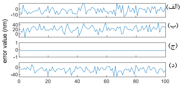
شکل ۱: اختلاف نتایج ناشی از الگوریتم کمترین مربعات نسبت به مقدار ایده‌آل شبیه‌سازی برحسب راه‌نوری در حضور: (الف) خطای لرزش با بیشینه ۲۰ نانومتر، (ب) خطای پایداری دامنه با بیشینه ۰٫۲، (ج) خطای انتقال فاز به میزان ۱۰٪ به ازای هر گام، (د) هم‌زمان خطاهای بخش‌های (الف)، (ب) و (ج) در شبیه‌سازی.
