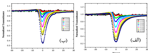
شکل ۳: نمودار تراگسیلندگی بهنجار عبوری جاروب محوری روزنه باز کادمیم تلوراید آلائیده شده با منگنز (الف) با ساخت چهار ساعت (ب) ساخت ۸ ساعت
