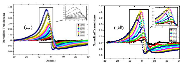
شکل ۴: نمودار تراگسیلندگی بهنجار عبوری جاروب محوری روزنه بسته کادمیم تلوراید آلائیده شده با منگنز (الف) با ساخت چهار ساعت (ب) ساخت ۸ ساعت
