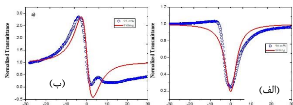
شکل ۲: نمودار تراگسیلندگی بهنجار عبوری جاروب محوری با برازش برای توان ۹۵ میلی‌وات کادمیم تلوراید آلائیده شده با منگنز با ساخت ۴ ساعت و برازش هر یک با استفاده از روابط (۵) و (۶)
