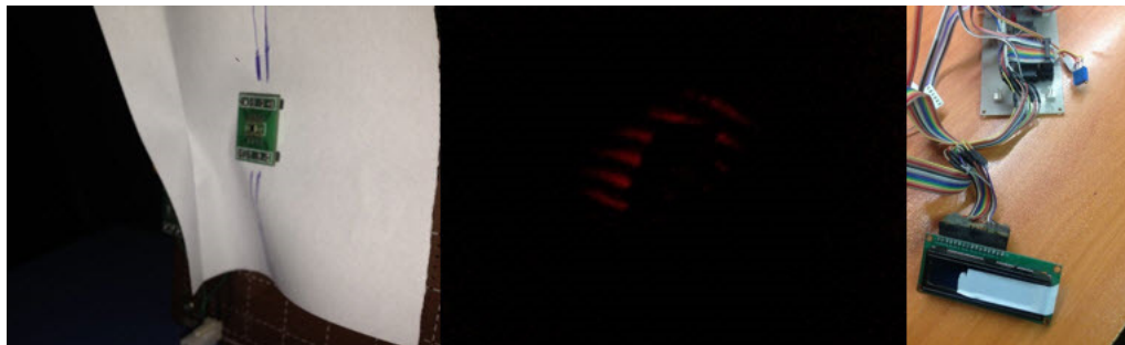
شکل ۲) تصویر مدارالکتریکی ساخته شده (سمت راست)، قرار فریزهای تداخلی گیری روی فتودیود (وسط)، موقعیت فتودیود بر روی پرده بدون تابش لیزر (سمت چپ)
