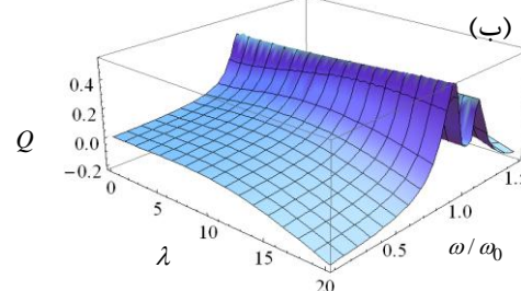
شکل ۴: پارامتر مندل برحسب \lambda و \omega/\omega_0 برای حالت همدوس غیرخطی خروجی از تیغه‌ی دی‌الکتریک مطابق پارامترهای شکل ۲.
