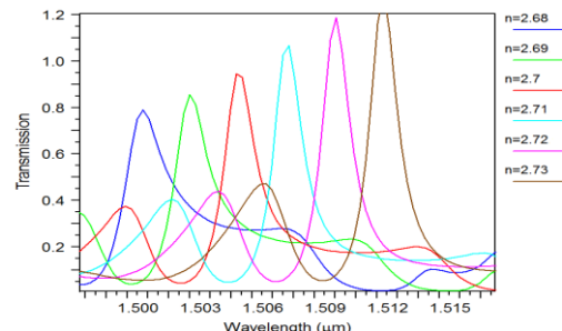
شکل ۵: اثر مقادیر مختلف n در روی ساختار فیلتر
