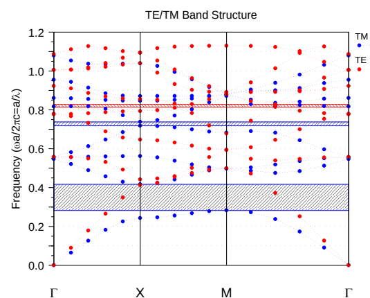
شکل ۱: ساختار باند کریستال فوتونیکی بکار رفته برای طراحی فیلتر
