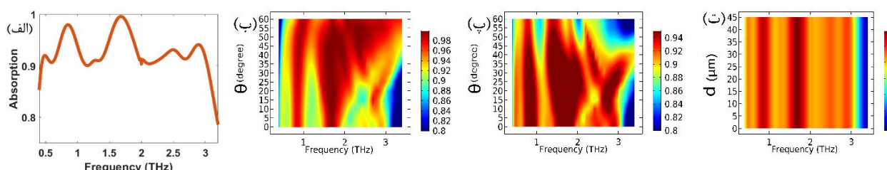
شکل ۲ (الف) ضریب جذب محاسبه شده برای ساختار در فاصله ۰/۴ تا ۳/۲ تراهرتز (ب) جذب به ازای زاویه‌های ۰ تا ۶۰ درجه برای قطبش TE (پ) جذب به ازای زاویه‌های ۰ تا ۶۰ درجه برای قطبش TM (ت) جذب به ازای تغییرات ناهمترای بین لایه‌ها
