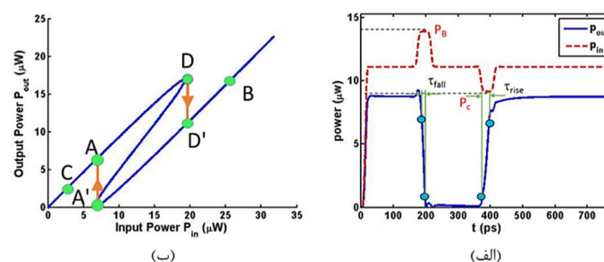
شکل ۱: (الف) نمودار تغییرات زمانی توان خروجی ساختار پیشنهادی به ازای شعاع میکرو-دیسک؛ R=0.92 \mu m ، (ب) نمودار توان خروجی ساختار تزویج شده موجبر و میکرو-دیسک بر حسب توان ورودی که نشان دهنده رفتار دوپایداری نوری در ساختار است.
