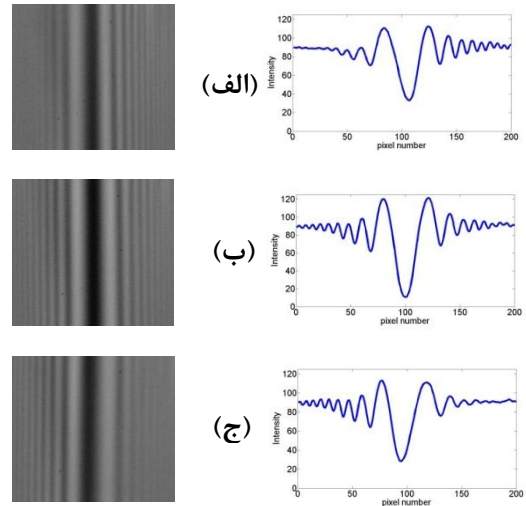
شکل ۲: نقش‌های پراش و نمایه های شدت آنها برای نور پراشیده از پله وقتی که اختلاف فاز الف) \varphi = (2m+1/2)\pi ، ب) \varphi = (2m+1)\pi (ج) \varphi = (2m+3/2)\pi است. m عدد صحیح است.
