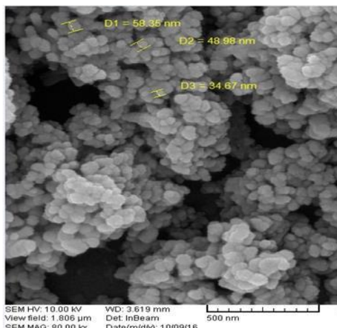
شکل ۵: ریخت‌شناسی اکسید روی آلاینده با نیکل.
