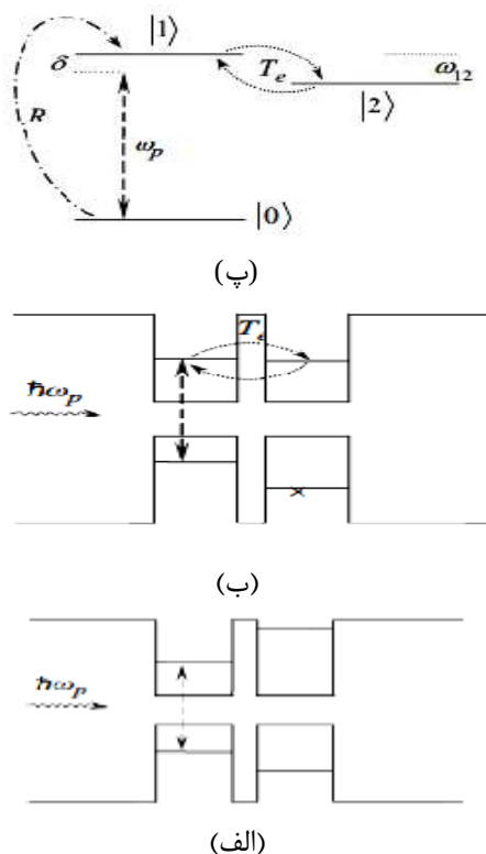
شکل ۲: ساختار نواری مولکول های نقاط کوانتومی (الف) قبل از اعمال ولتاژ گیت (ب) بعد از اعمال ولتاژ گیت (پ) ترازهای انرژی بعد از اعمال میدان کاوشگر
