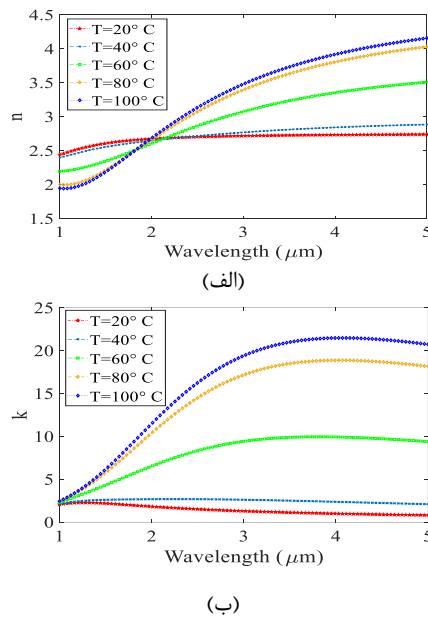
شکل ۲: قسمت‌های (الف) حقیقی و (ب) موهومی ضریب شکست VO_2 در دماهای مختلف.
