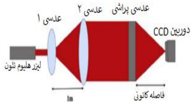
شکل ۴: چیدمان آزمایش
