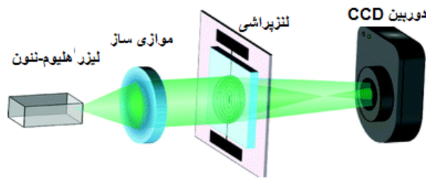
شکل ۳: چیدمان آزمایشگاهی
