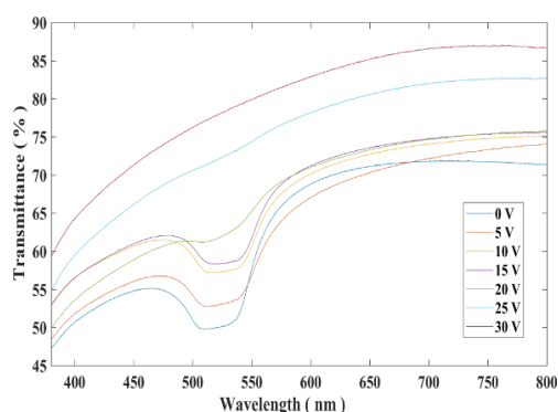
شکل (۴): جابجایی بازتاب براگ و تغییرات عبور نور برای نمونه ی بلورماید کستریک در حضور میدان الکتریکی خارجی
