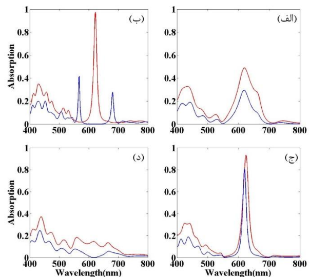
شکل ۴: طیف جذب (الف) و (ب) ساختارهای ADPC به ترتیب با ضخامت نقص نیم موج و ربع موج (ج) و (د) ساختارهای SDPC به ترتیب با ضخامت نقص نیم موج و ربع موج. در تمامی شکل‌ها رنگ قرمز و آبی به ترتیب برای نقص MDM و DMD می‌باشد.
