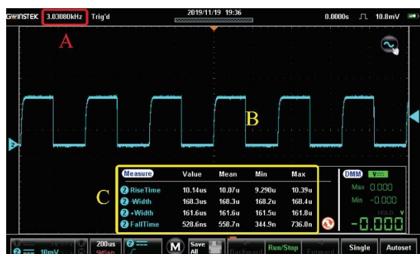
شکل ۳: نمایی از خروجی اسیلوسکوپ دیجیتال متصل به حسگر فوق سریع (A): فرکانس قطار پالس لیزر، (B) نمای پالس مدوله شده روی لیزر دیودی، (C) اطلاعات مربوط به پالس همچون پهنا و زمان خیز/افت.
