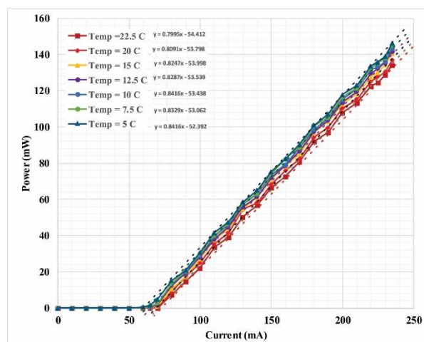
شکل ۳: نمودار جریان-توان لیزر دیودی در دماهای متفاوت
