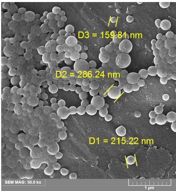
شکل ۱: تصویر میکروسکوپ الکترونی روبشی گسیل میدانی از نانوکپسول‌های تهیه شده با پوسته پلیمری و هسته بلورمایع دوپه شده با رنگینه.
