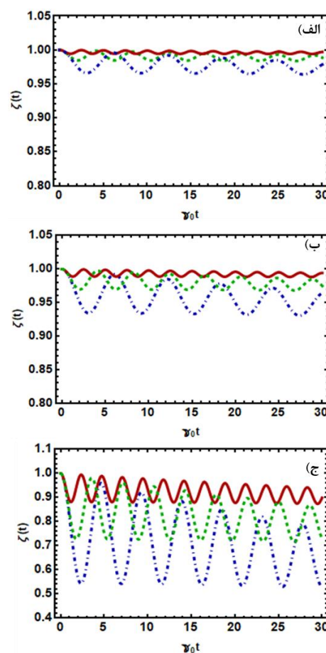
شکل ۲: همدوسی بر حسب زمان مقیاس شده به ازای پارامترهای G = 4\gamma_0 , \delta = 3.6\gamma_0 , \Omega = 5\gamma_0 , \lambda = 0.01\gamma_0 (نقطه خط آبی)، G = 2.5\gamma_0 (خط پیوسته قرمز) و G = 6.5\gamma_0 (خط چین سبز) که در حضور الف) گذار تک فوتونی، ب) دوفوتونی و ج) چهارفوتونی رسم شده است.
