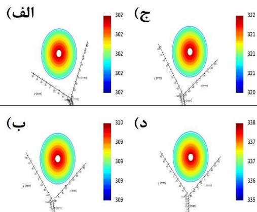
شکل ۲: دمای مقطع عرضی کندکننده زیمان در زمانی که تبادل حرارتی مجموعه با محیط به تعادل رسیده است به ترتیب برای جریان‌های الف) ۰/۵ (ب) ۱ (ج) ۱/۵ و د) ۲ آمپر
