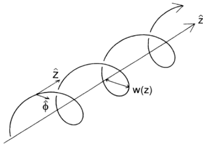
شکل ۱) منحنی ماریچی بردار پویینتینگ برای باریکه‌ی لاگر-گوسی [۸].
