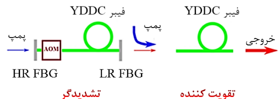
شکل ۱: طرح لیزر فیبری سوئیچ Q؛ در شکل: AOM: آلان آکوستو اپتیک، FBG: تار نوری براگ
