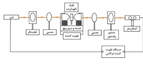
شکل ۱: طرحواره‌ی از چیدمان فارادی.
