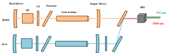
شکل ۵: طرحواره ای از لیزر Master-Slave
