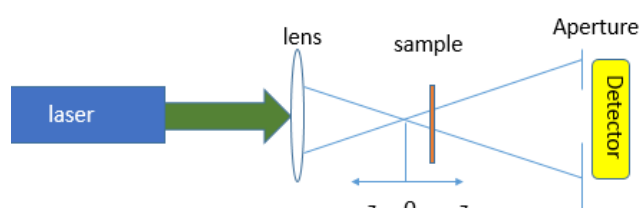
شکل ۱: شماتیک چیدمان جاروب Z روزنه بسته
