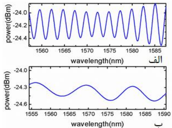
شکل ۴ اعمال فیلتر میان گذر برای جدا کردن طیف طول موج دو کاواک (الف) کاواک 370 \mu\text{m} (ب) کاواک 80 \mu\text{m}
