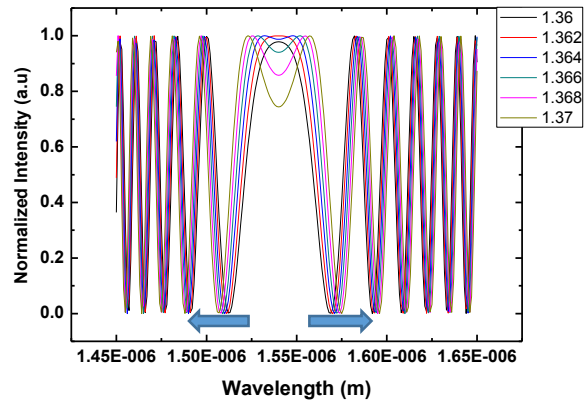
شکل ۲: نمودار جایجایی طول موجی طیف تداخلی با تغییر ضریب شکست محیط خارجی در بازه ی ۱,۳۶ تا ۱,۳۷
