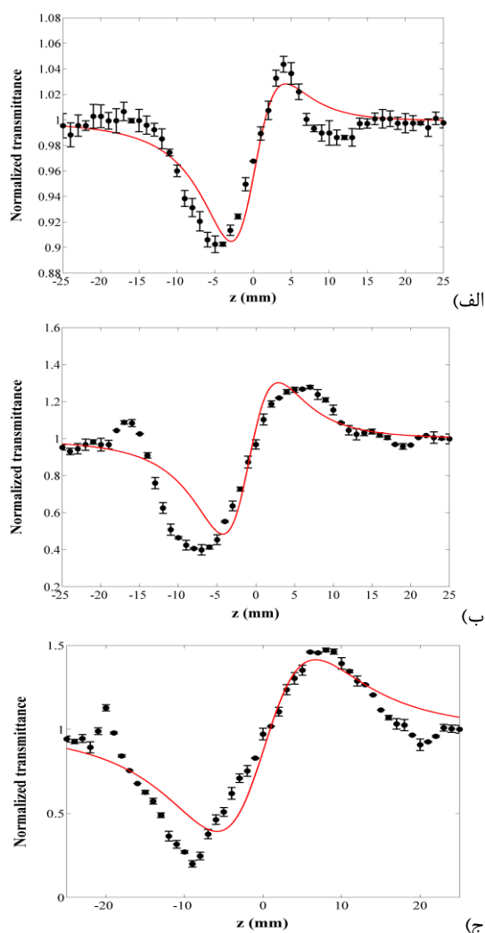
شکل ۳. داده های رویش Z روزنه بسته (نقاط) و برازش (خط قرمز) برای نمونه های الف) \text{PS-2\% TiO}_2 ، ب) \text{PS-4\% TiO}_2 و ج) \text{PS-6\% TiO}_2 .
