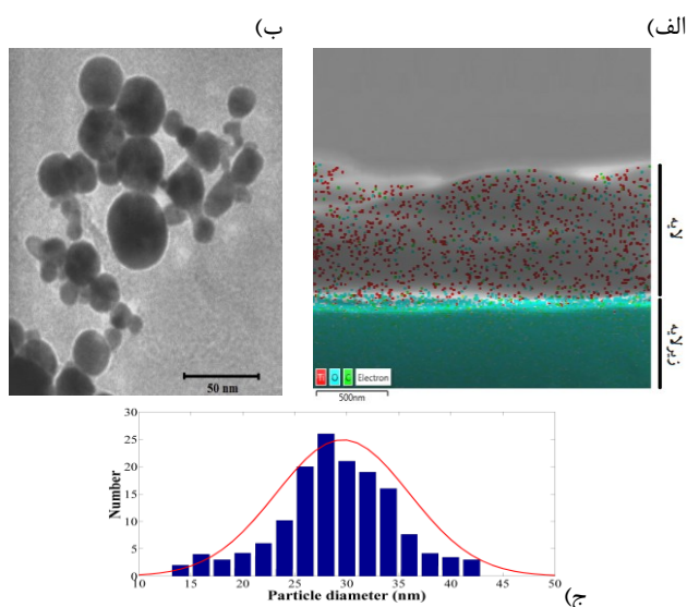
شکل ۲. الف) تصویر SEM سطح مقطعی لایه نانوکامپوزیت PS-6% TiO2. ب) تصویر میکروسکوپ الکترون عبوری نانوذرات و ج) توزیع اندازه نانوذرات.
