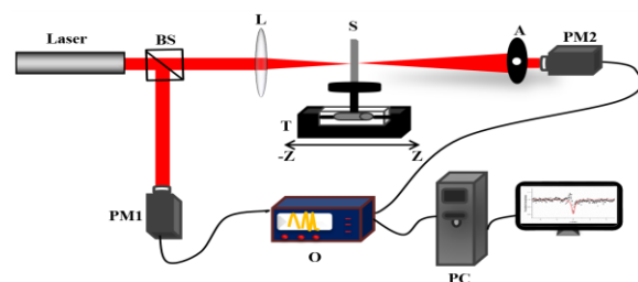
شکل ۱: طرح چیدمان آزمایشگاهی روبش Z روزنه بسته. BS: شکافنده باریکه مکعبی، L: عدسی، S: نمونه لایه نازک، A: روزنه، PM1 و PM2: توان سنج، T: جابه‌جاگر نمونه.
