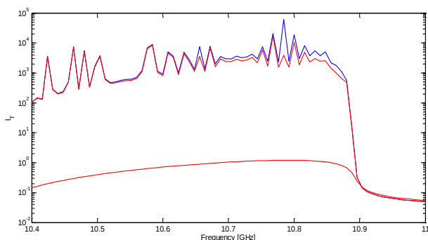
شکل ۳: طول تراگسیل l_T بر حسب فرکانس f در حالت \theta_a = 30^\circ برای یک ساختار متماده، بدون حضور جذب و با قطبش p (منحنی آبی رنگ) و با قطبش s (منحنی قرمز رنگ) و در حضور جذب (منحنی پایینی).
